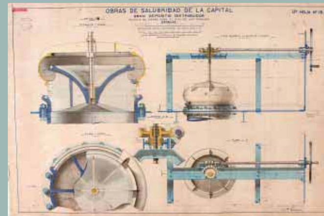
Gran depósito distribuidor. Plano de valvula de cierre, 1899.
